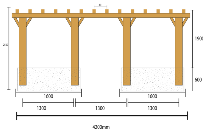
Prototype stadspergola: zij aanzicht
