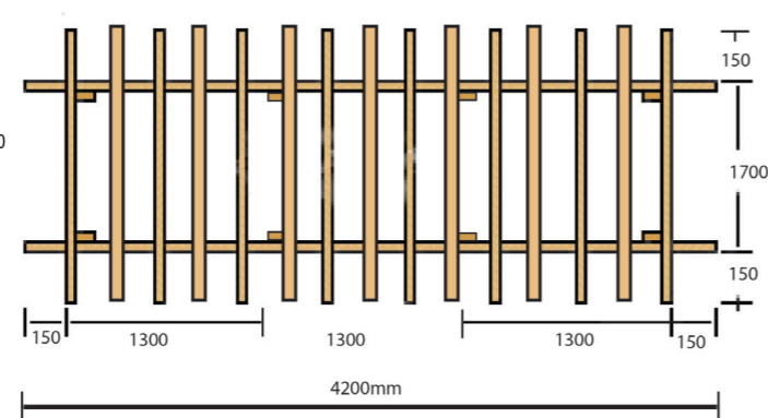
Prototype stadspergola: bovenaanzicht
