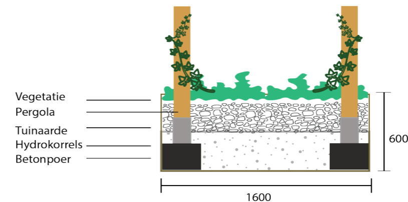
Prototype stadspergola: doorsnede plantenvak en bevestiging
